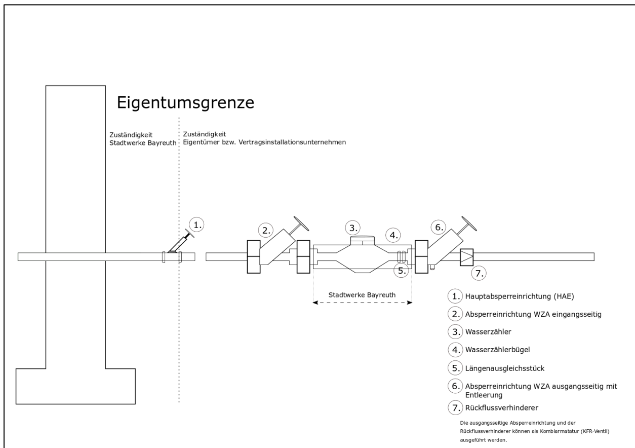
Abbildung 1: Hausanschluss Eigentumsgrenze
